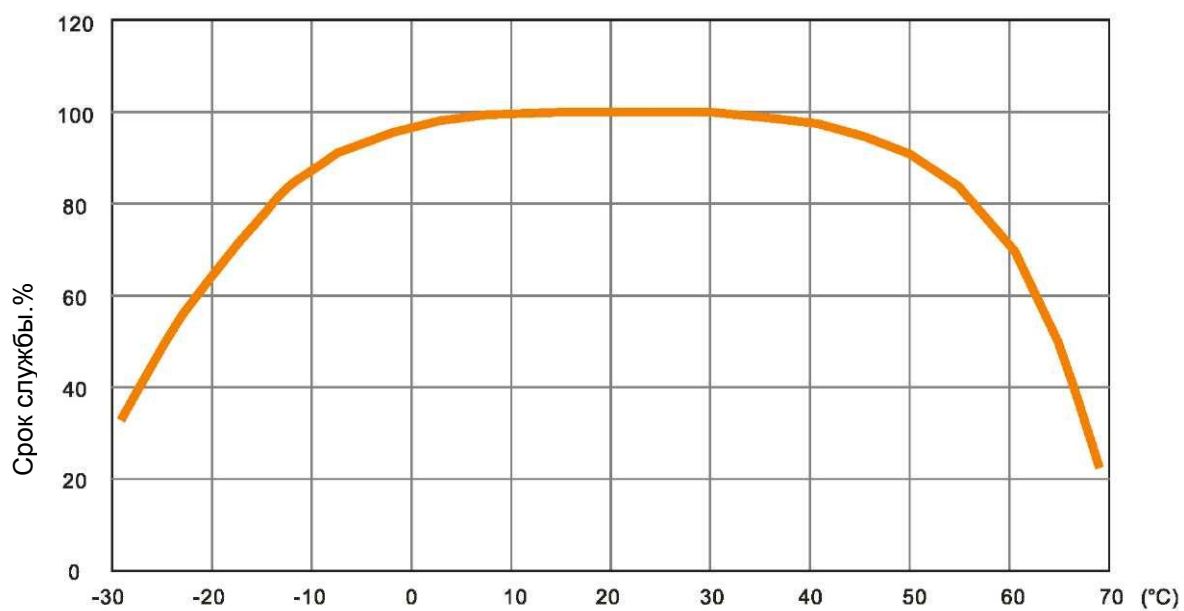
Относительная зависимость (%) срока службы от окружающей температуры
