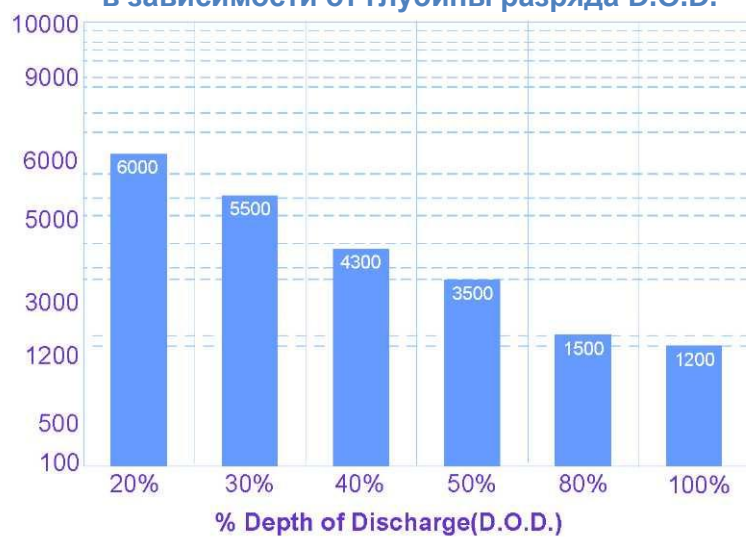
Циклический ресурс аккумуляторов OPzS в зависимости от глубины разряда D.O.D.
