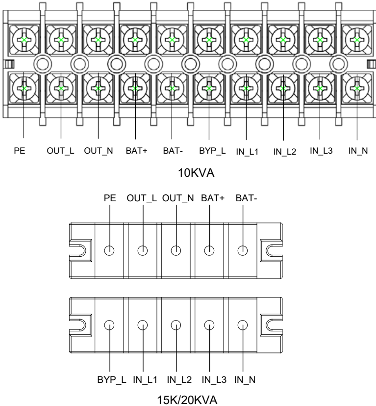
Рис. 2-1: Схема підключення клемної колодки
