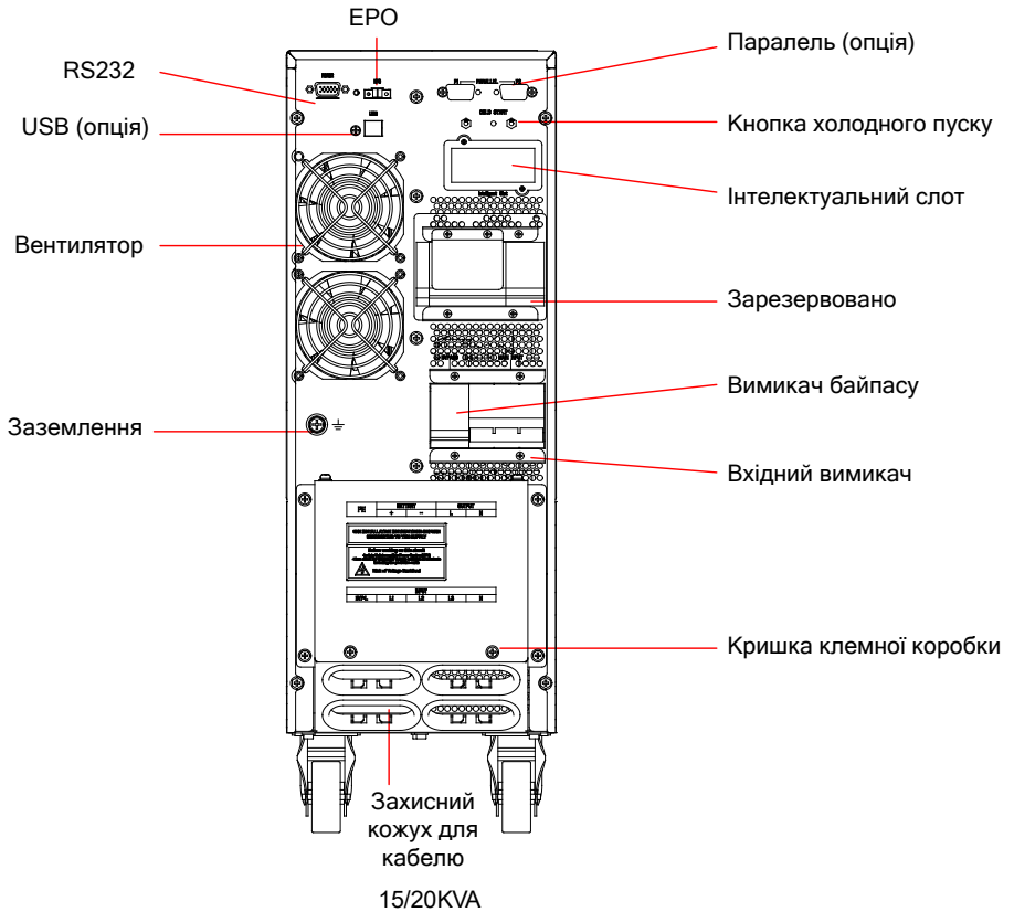
Рис 1-2: Вид ззаду
