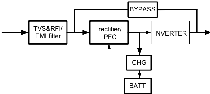
Рис. 1-5: Режим байпасу
