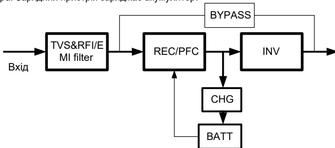
Рис 1-4: Нормальний режим
