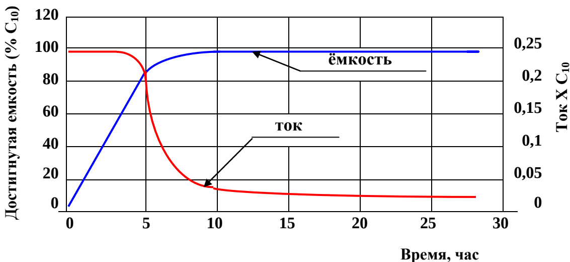
Зарядка после полной разрядки с токоограничением 0.25C_{10} А и напряжением 2.30 В /элемент
