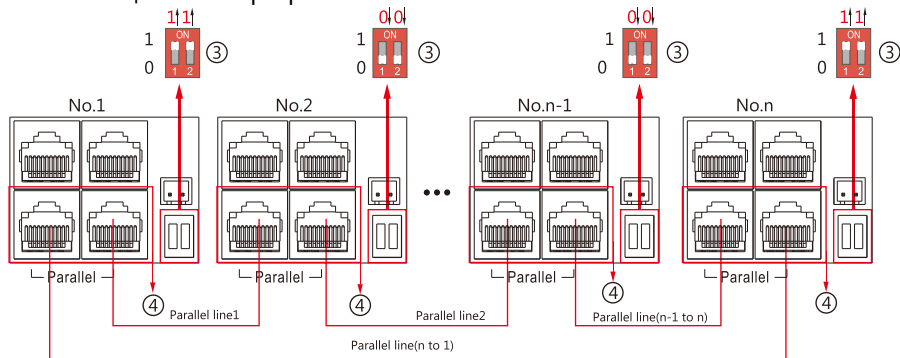
Максимальна кількість підключених інверторів 10, отже 2 < n < 10
