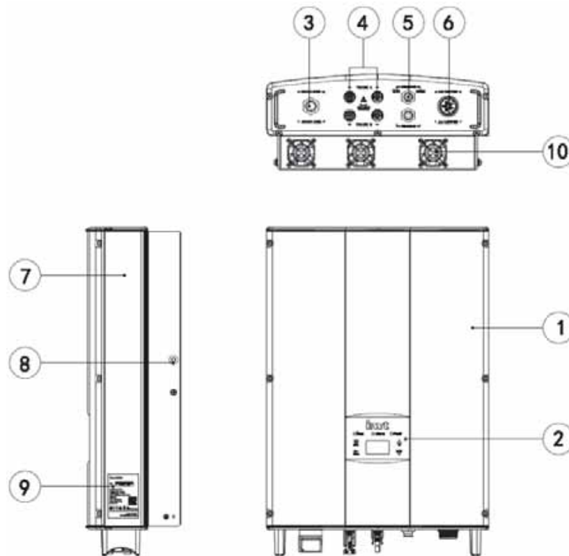
Рисунок 2.3 Внешний вид инвертора
