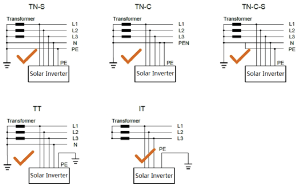
Рисунок 2.2 Типы сети
