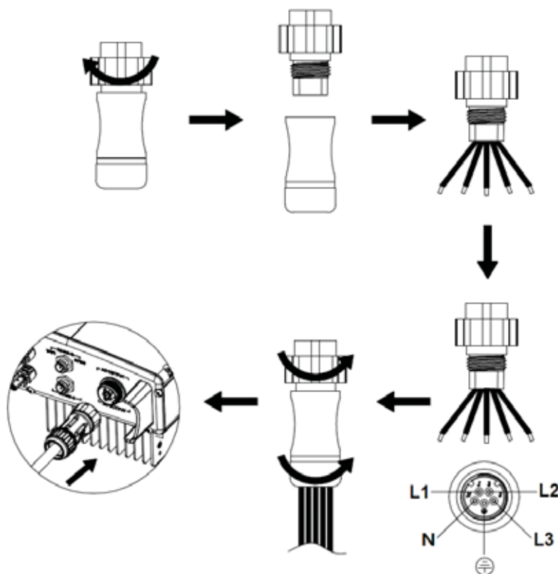
Рисунок 4.13 Подключение переменного тока к трёхфазному инвертору
