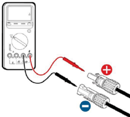
Рисунок 4.12 Измерение входного напряжения постоянного тока
