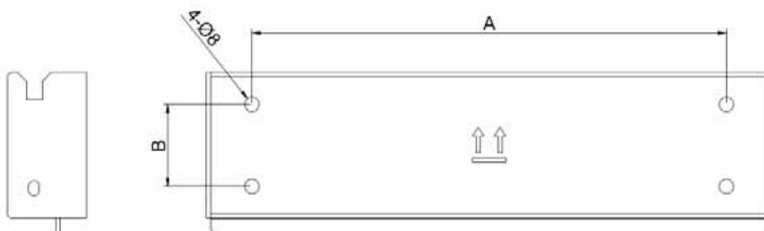
Рисунок 4.3 Монтажный кронштейн для инвертора 6~12 кВт
