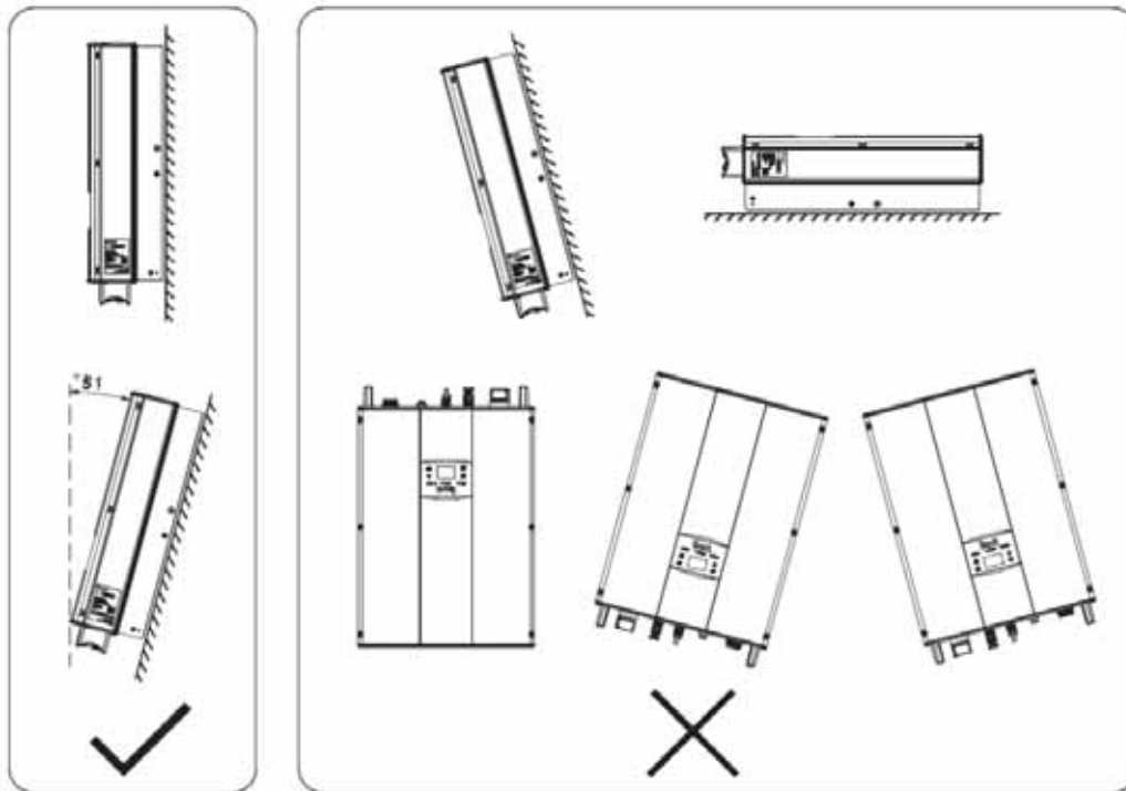
Рисунок 4.2 Положение установки инвертора
