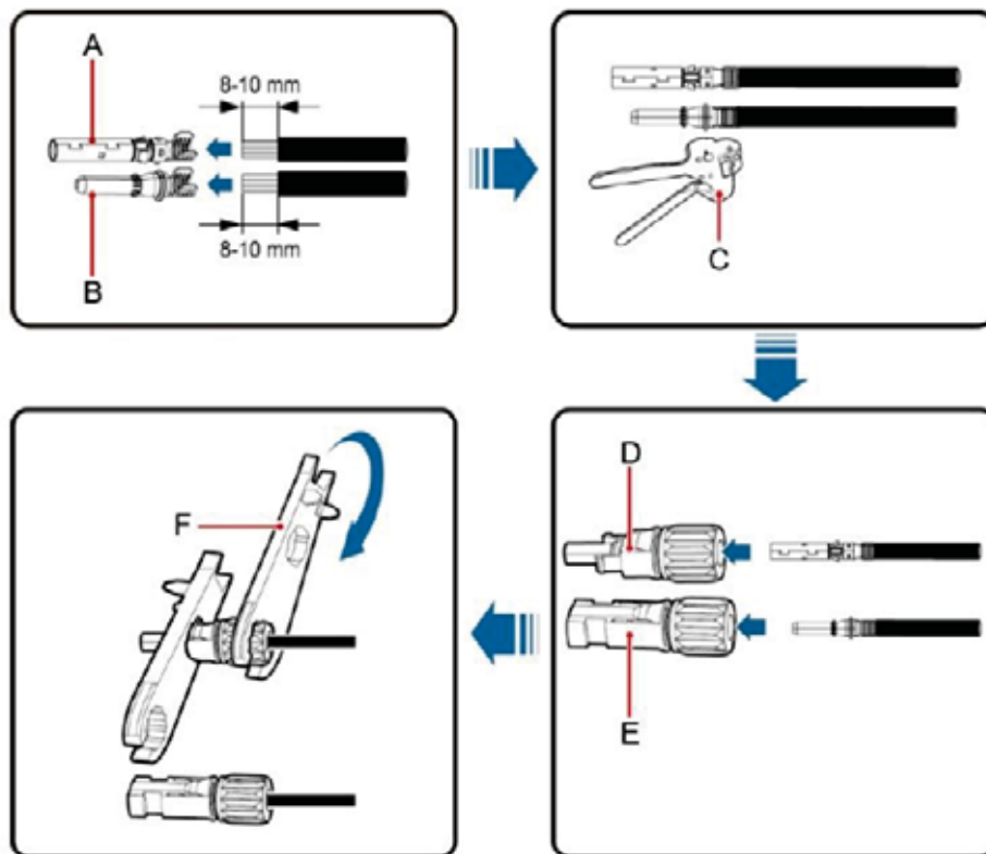
Рисунок 4.11 Соединение между разъемом постоянного тока и солнечными модулями
