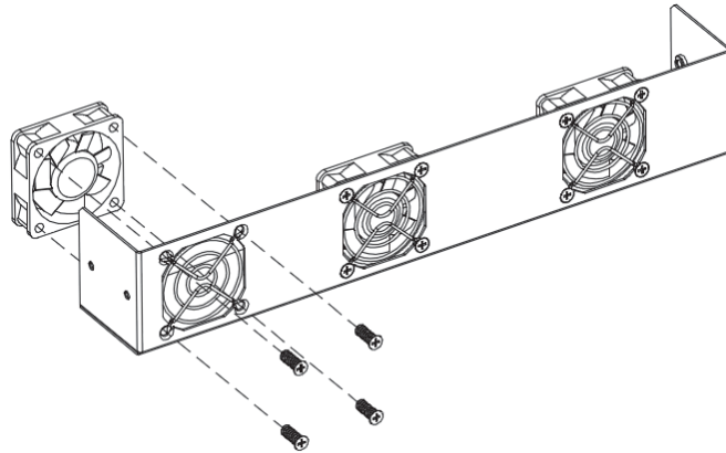
Рисунок 5.3 Снимите вентилятор
