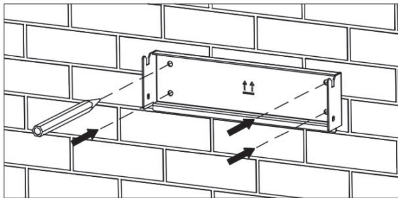
Рисунок 4.4 Отметьте места для отверстий
