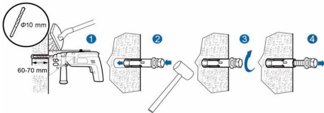
Рисунок 4.6 Установка дюбелей
