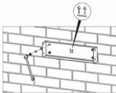
Рисунок 4.7 Закрепите монтажный кронштейн
