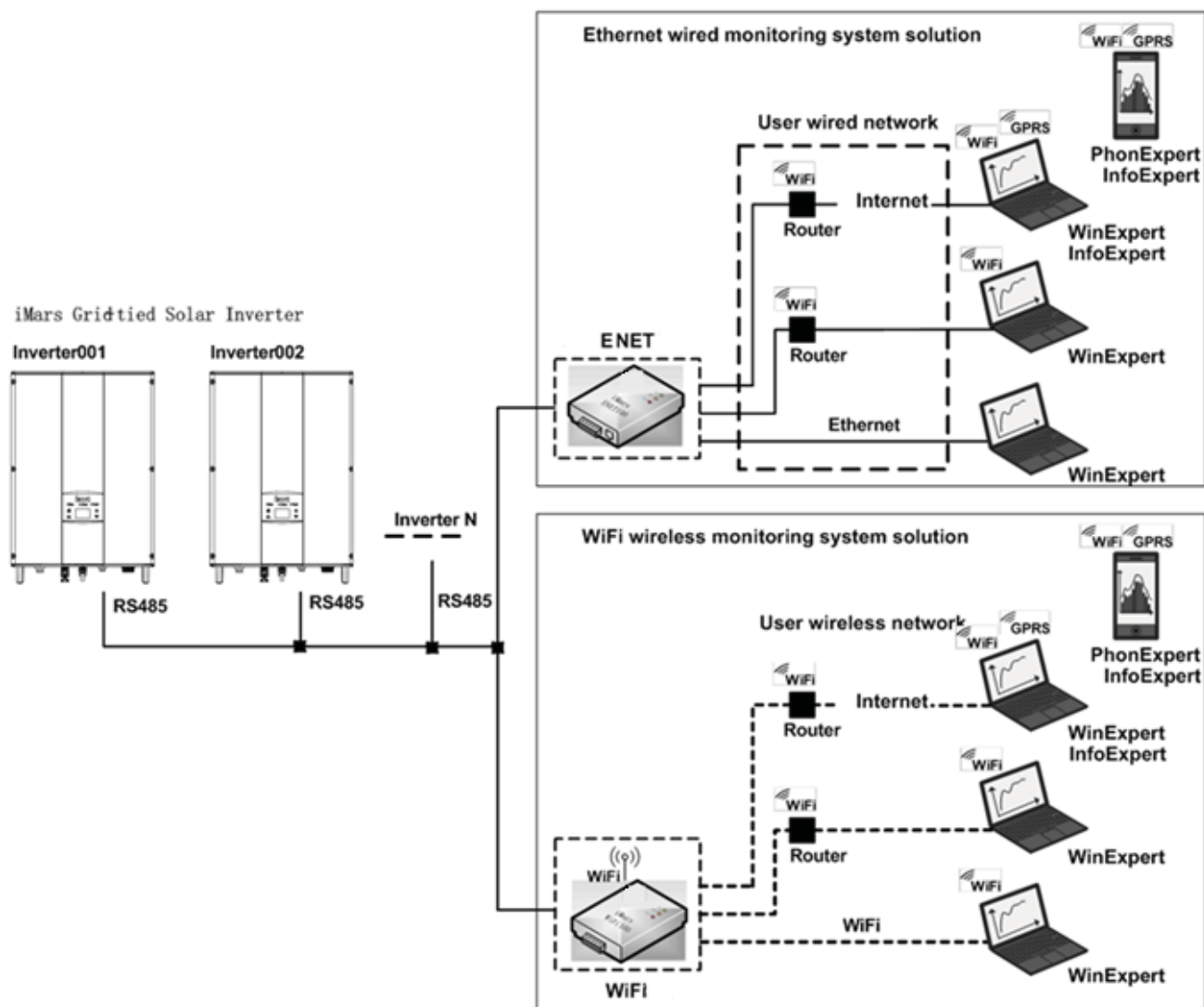
Рисунок 7.1 Система мониторинга инвертора
