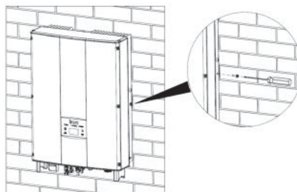
Рисунок 4.9 Затяните болты М5Х20
