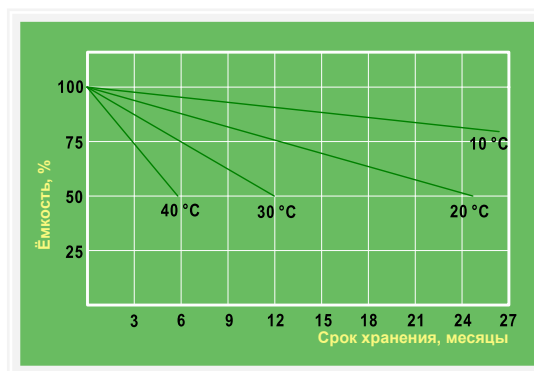
Саморазряд при различных температурах окружающей среды
