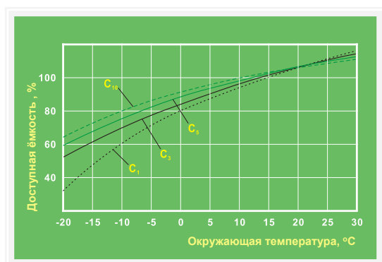
Ёмкость в зависимости от окружающей температуры
