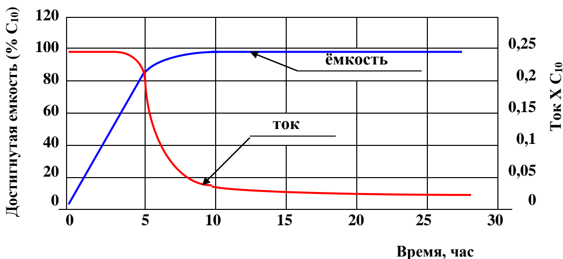
Зарядка после полной разрядки с токоограничением 0.25C_{10} А и напряжением 2.30 В /элемент
