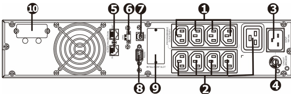
Рисунок 3. Задняя панель ИБП CORE 3К
