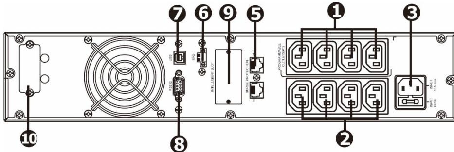
Рисунок 1. Задняя панель ИБП CORE 1К
