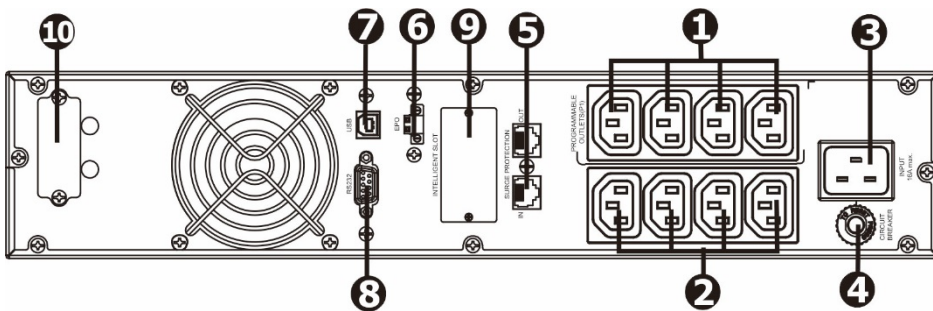
Рисунок 2. Задняя панель ИБП CORE 2К
