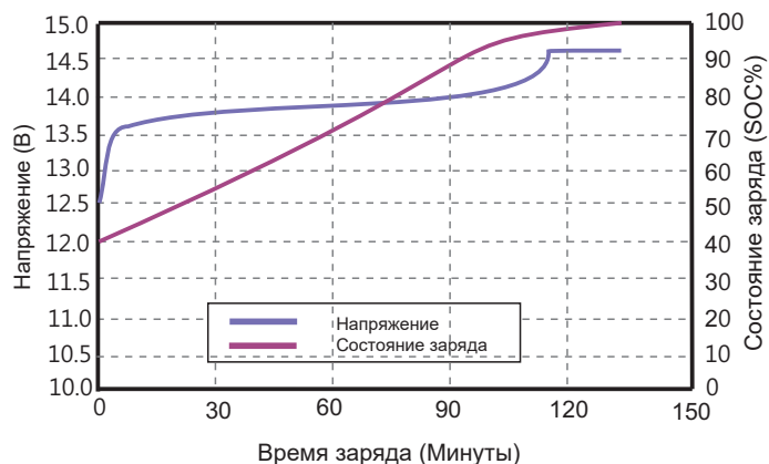
Кривая состояния заряда при 0,5C 25°C
