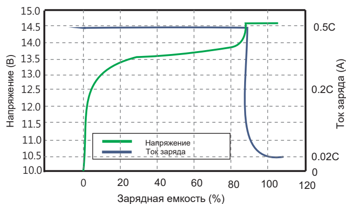
Зарядные характеристики при 0,5C 25°C
