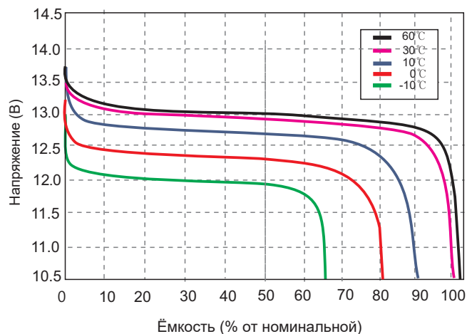
Кривые разряда при различных температурах при 0.5C
